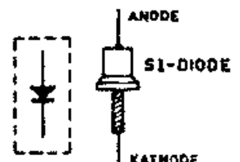
ANODE S1-DIODE KATHODE 0A 214 G 501
