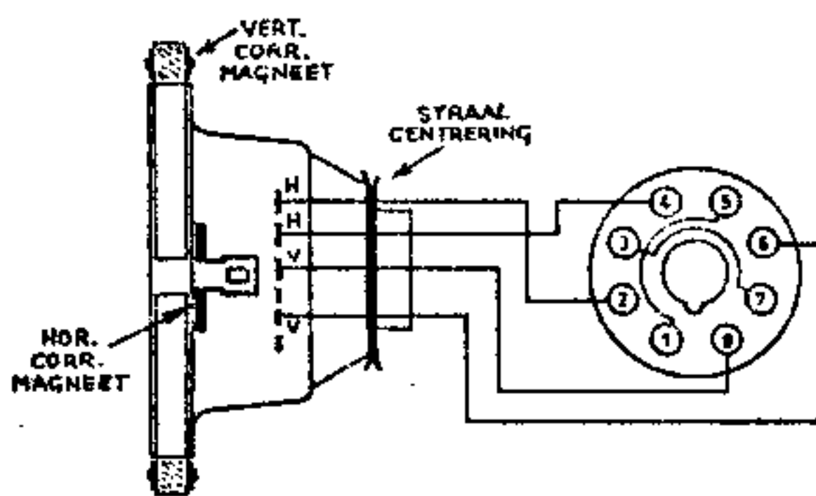
DEFLECTIE JUK DEFLECTION YOKE ABLENKEINHEIT AT 1009/02
